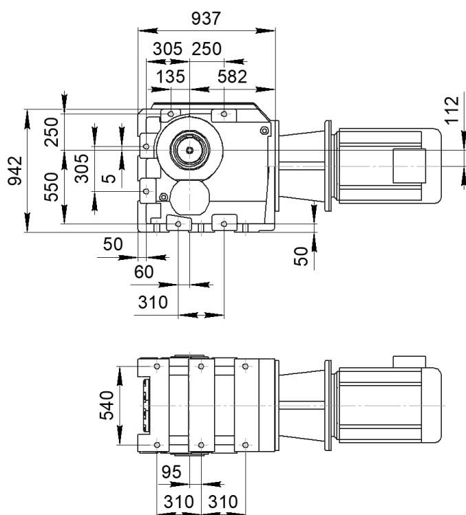
РАЗМЕРЫ ЦИЛИНДРИЧЕСКОГО ВЫХОДНОГО ВАЛА K, KF
