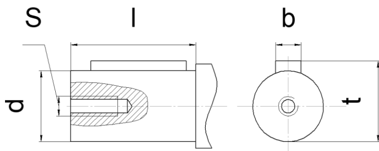
РАЗМЕРЫ ЦИЛИНДРИЧЕСКОГО ВЫХОДНОГО ВАЛА K, KF
